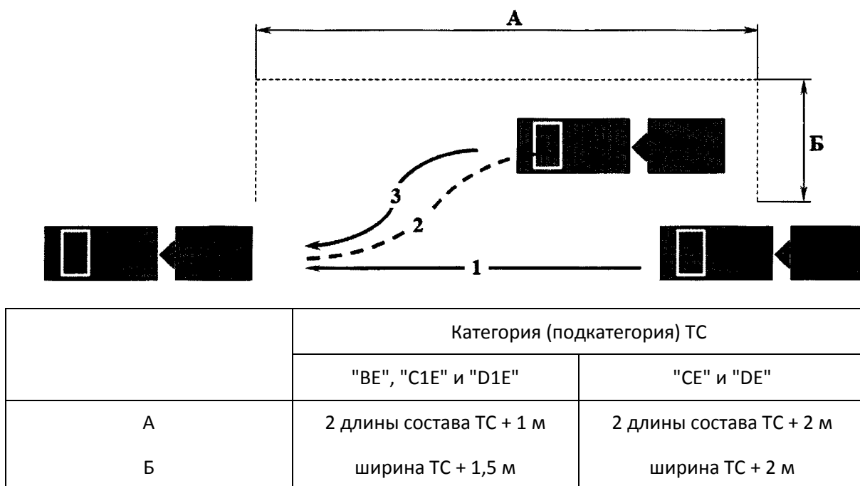
Рисунок 5. Схема и размеры маневра "Постановка транспортного средства на место стоянки параллельно тротуару (краю проезжей части) при движении задним ходом"
