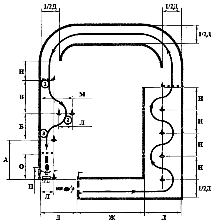
Рисунок 5. Схема "Б" упражнения N 4.
