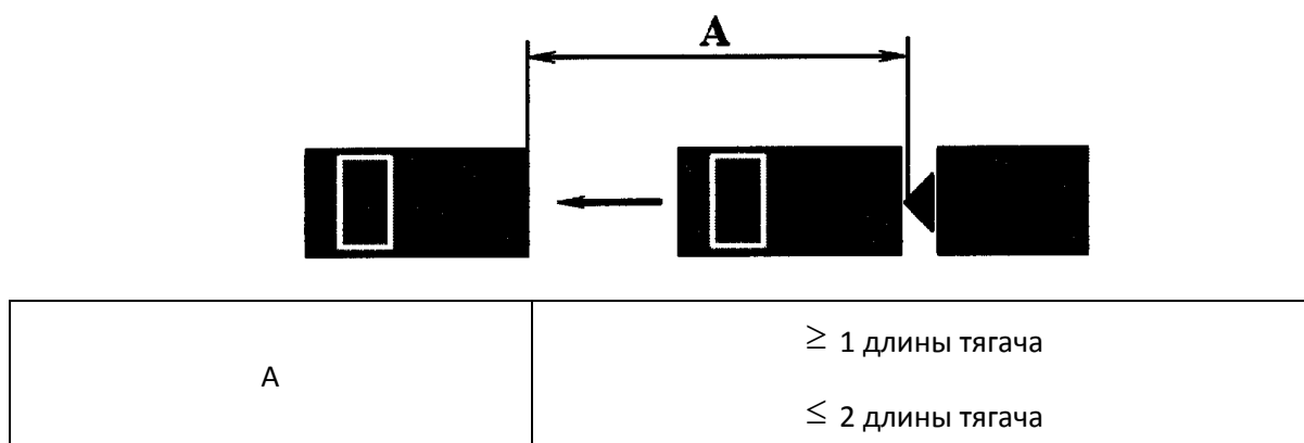
Рисунок 8. Схема и размеры маневра "Сцепление и расцепление или расцепление и повторное сцепление прицепа с тягачом (для транспортных средств категорий "BE", "CE" и "DE" и подкатегорий "C1E" и "D1E", за исключением сочлененных автобусов)" при расцеплении прицепа с тягачом
