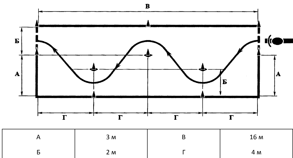
Рисунок 3. Схема и размеры упражнения N 3
