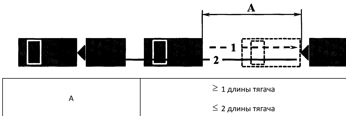
Рисунок 9. Схема и размеры маневра "Сцепление и расцепление или расцепление и повторное сцепление прицепа с тягачом (для транспортных средств категорий "BE", "CE" и "DE" и подкатегорий "C1E" и "D1E", за исключением сочлененных автобусов)" при сцеплении прицепа с тягачом
