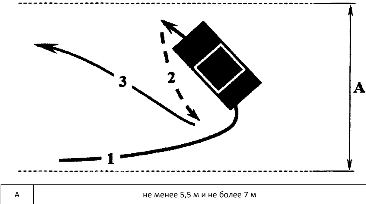
Рисунок 7. Схема маневра "Разворот транспортного средства в ограниченном пространстве (при ограниченной ширине проезжей части) с использованием движения задним ходом"
